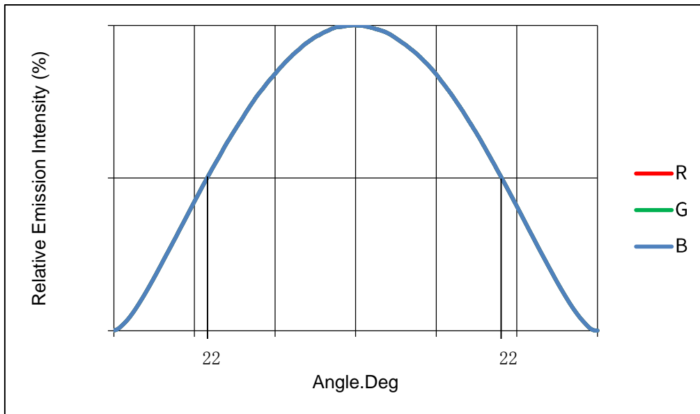
Fig 1-11 Directivity X-X radiation angle X轴方向輻射角度
